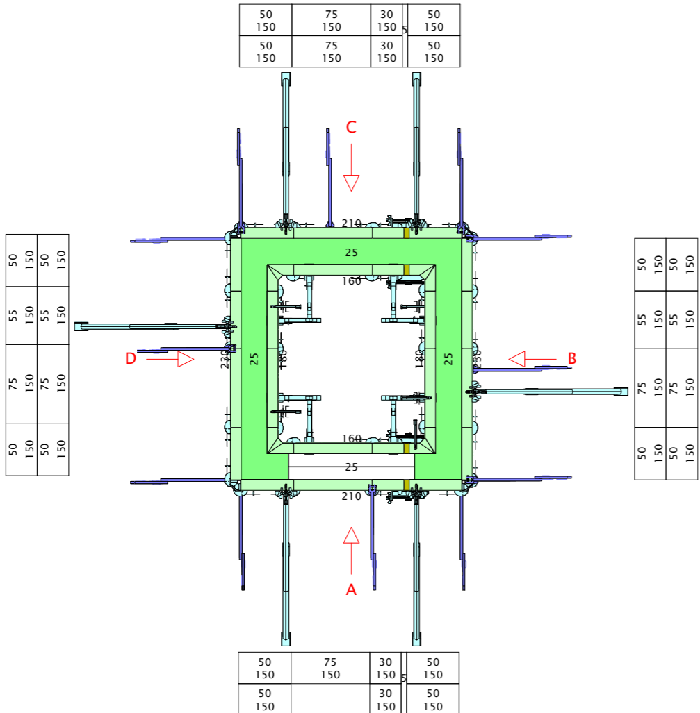
Grundriss 1:25
